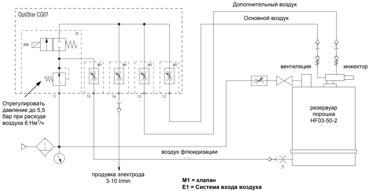
Пневматическая диаграмма - OptiFlex F
